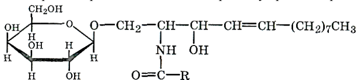
галактоцереброзиды (R – углеводородный радикал).
